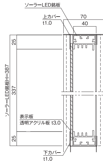
B-B'断面図 (S=1:4)
