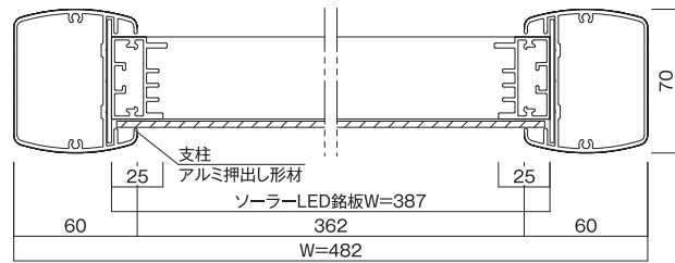
A-A'断面図 (S=1:4)
